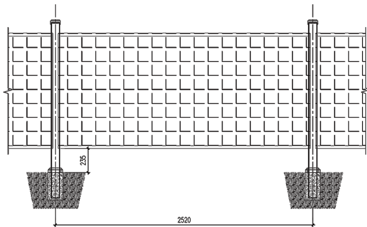
665W光伏围墙立面
