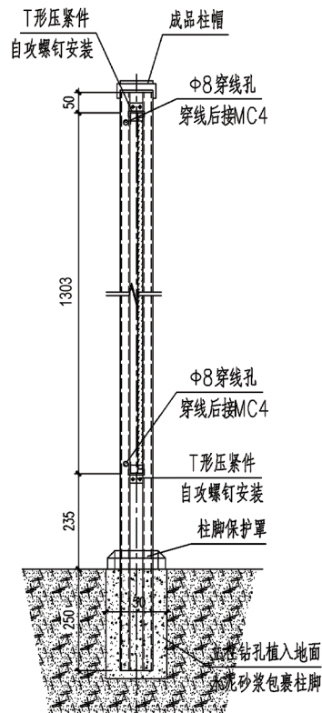
组件与立柱固定方式
