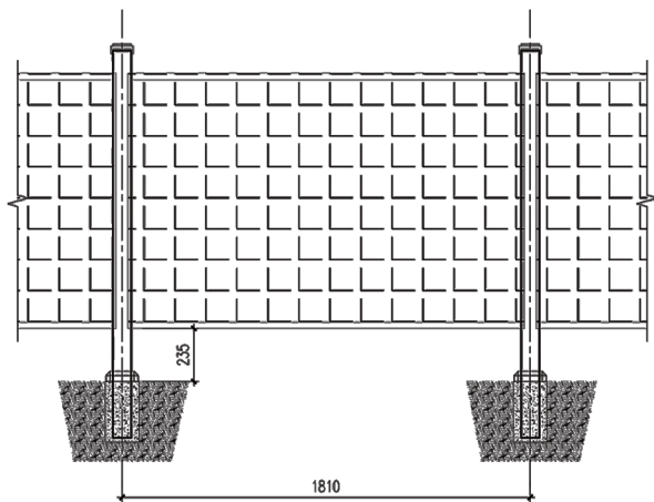
450W光伏围墙立面
